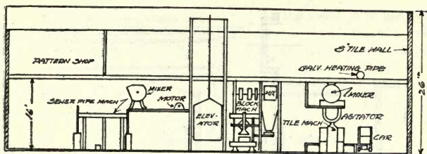
— SECTIONAL ELEVATION A. B. —
